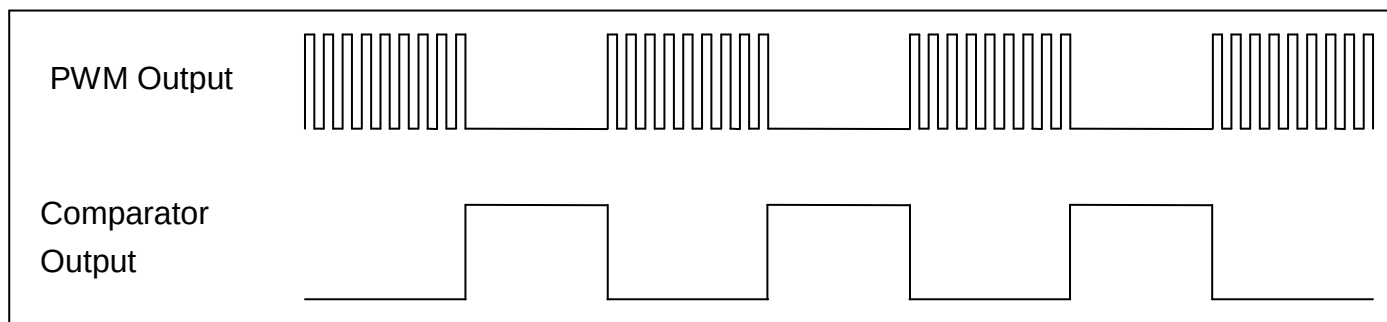
图 12: 比较器控制 PWM 波形的输出
