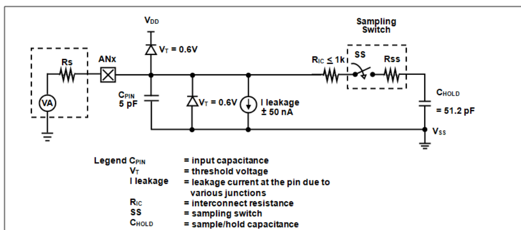
图 19：模拟输入模型
