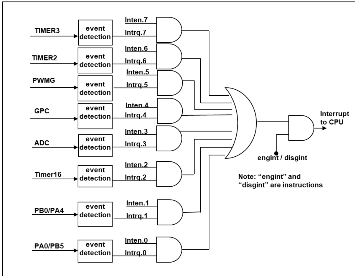
图 16: 中断控制器硬件框图
